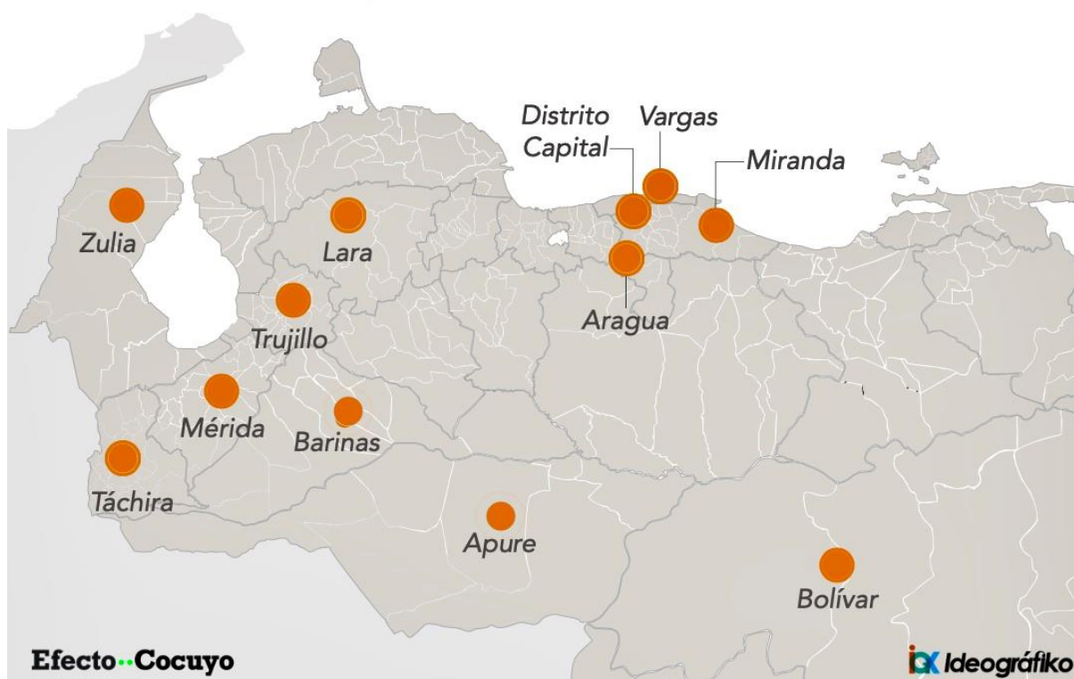
Karte 7: Präsenz der „Friedensmannschaften“ oder cuadrillas de paz , die auch als colectivos bekannt sind, in Venezuela, 7. April 2019 © Efecto Cocuyo/Ideografiko 1055
